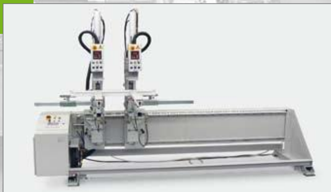
Soldadora de dos cabezales AKS 5600/2
